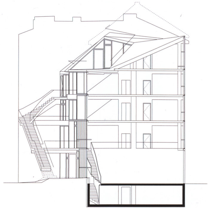
SECCIÓN DEL EDIFICIO. SECTION OF THE BUILDING.
